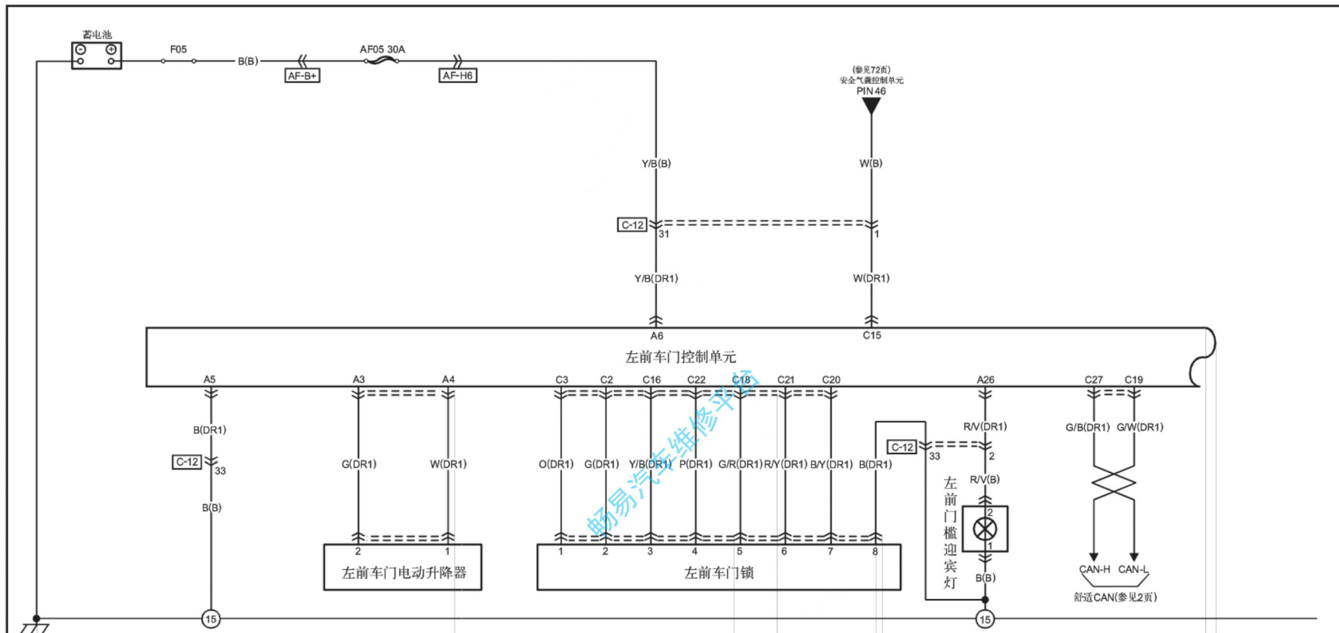
左前车门控制单元A
